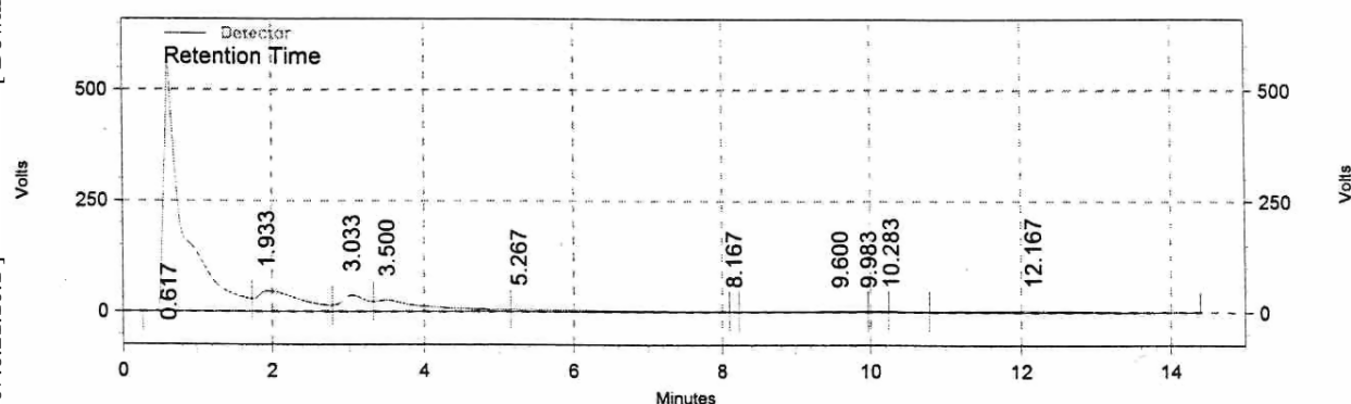
شکل شماره ۳ - کروماتوگرام نمونه مورد آنالیز برگ جینکو بایلوپا
