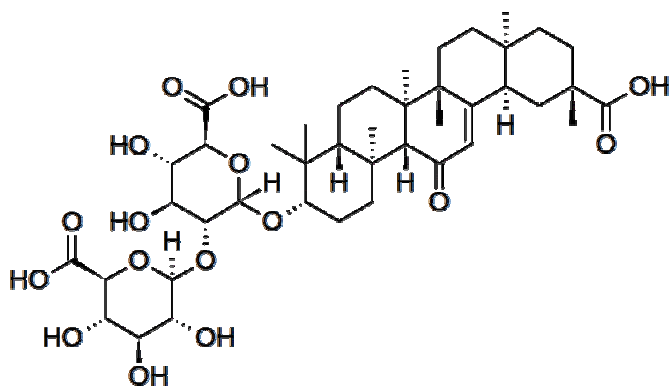
Fig. 1- Glycyrrhizin
