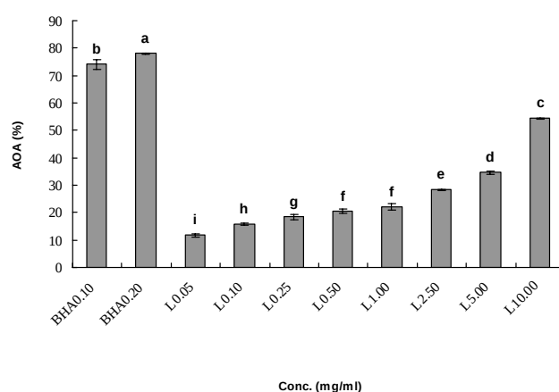
شکل شماره ۲- مقایسه‌ی فعالیت ضداکسایشی اسانس اسطوخودوس با ضداکساینده سنتزی BHA توسط آزمون بی رنگ شدن بتاکاروتن. نتایج میانگین سه تکرار \pm انحراف معیار است. حروف مختلف بیانگر اختلاف معنی دار در سطح ۹۵ درصد است.
