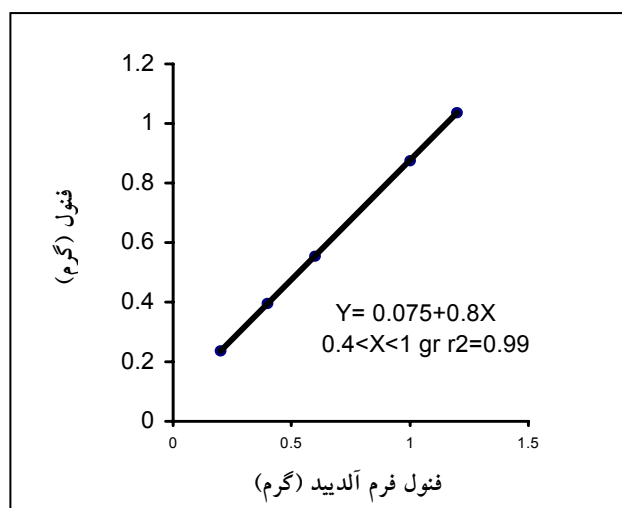
نمودار شماره ۱- منحنی رگرسیون بین فنول و رزین فنول - فرم آلدیید
