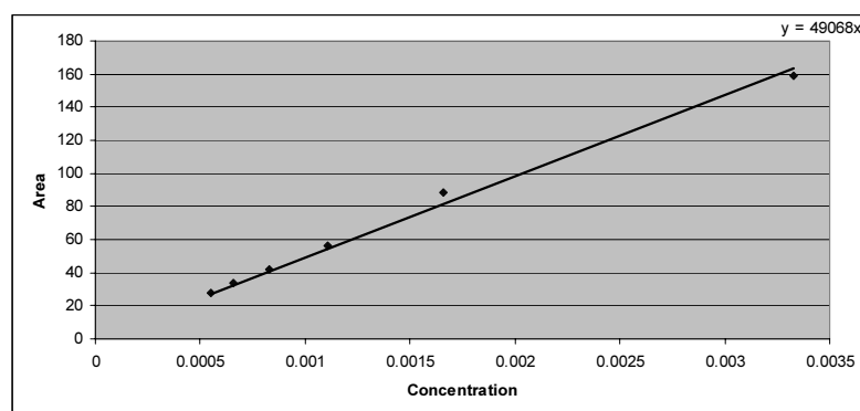
شکل شماره ۲ - منحنی کالیبراسیون ترکیب کوئرتستین
