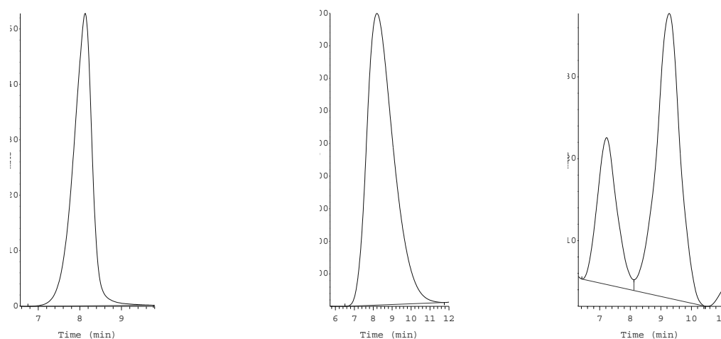
شکل شماره ۳- کروماتوگرام استاندارد کوئرستین و کمرول و نمونه گلبرگ گل محمدی
