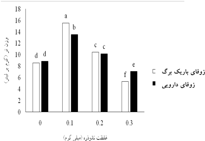
شکل ۳. مقایسه میانگین وزن تر در دو گونه زوفا تحت تأثیر تیمارهای مختلف نانوذرات نقره
