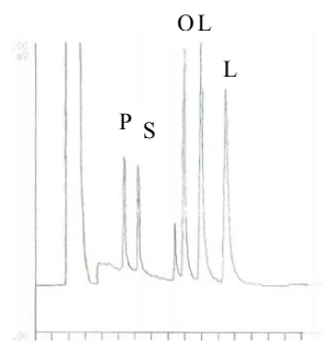
شکل شماره ۱۰ - کروماتوگرام متیل استر اسیدهای چرب روغن فراسودمند تولید شده با استفاده از دستگاه GC اسید پالمیتیک: p اسید استئاریک: S اسید اولئیک: O اسید لینولئیک: L اسید لینولئیک (Ln):
