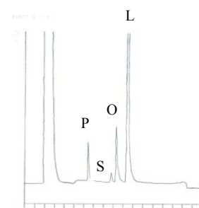
شکل شماره ۶- کروماتوگرام متیل استر اسیدهای چرب گلرنگ
