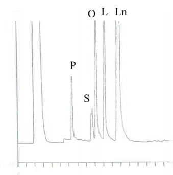
شکل شماره ۹- کروماتوگرام متیل استر اسیدهای چرب روغن بزرک در مرحله آخر جزء به جزء سازی با استفاده از دستگاه GC اسید لینولئیک: L اسید لینولئیک (Ln):
