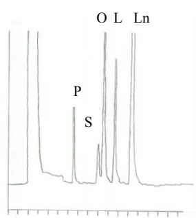
شکل شماره ۷- کروماتوگرام متیل استر اسیدهای چرب بزرگ
