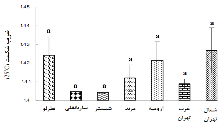
شکل شماره ۳- میزان ضریب شکست روغن کرچک در مناطق مختلف کاشت
