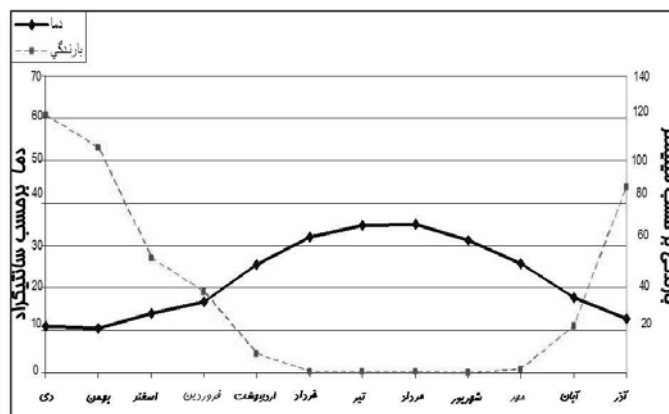
شکل شماره ۲- منحنی دما - باران شهرستان کازرون - طول مقطع بین دو منحنی طول دوره خشکی و دامنه آن شدت دوره خشکی منطقه را نشان می‌دهد [برگرفته از دولخواهی و همکاران [۹]]
