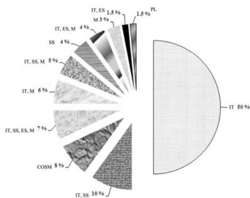
شکل شماره ۵- پراکنش جغرافیایی گونه های گیاهی دارویی منطقه کازرون - علائم اختصاری جغرافیای گیاهی: ایران- تورانی=IT؛ صحرا- سندی=SS، اروپا- سبیری=ES؛ مدیترانه ای=M؛ جهانی=COSM؛ چند ناحیه ای=PL
