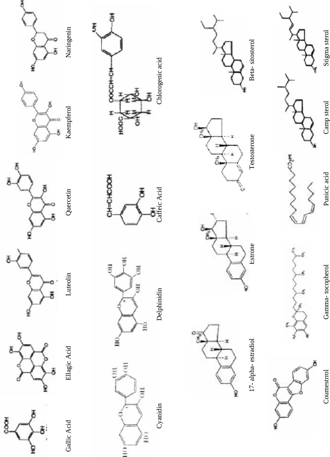
شکل شماره ۱ - ساختار شیمیایی برخی از ترکیبات شناسایی شده در میوه انار
