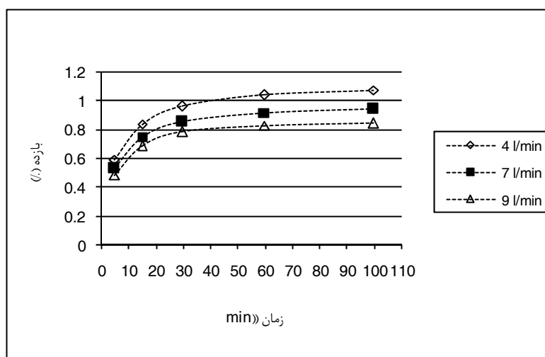
شکل شماره ۲- تغییرات بازده استخراج روغن‌های فرار نسبت به تغییرات شدت جریان حجمی بخار
