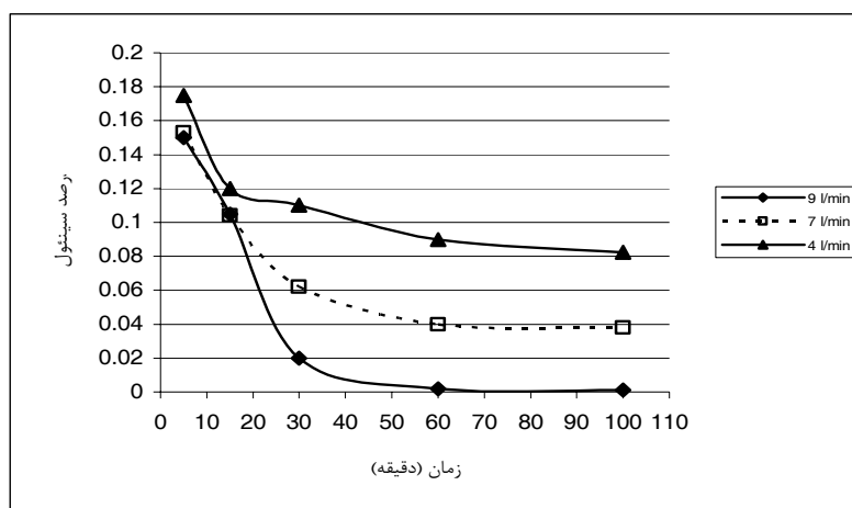
شکل شماره ۷- تغییرات ۱,۸- سینثول نسبت به زمان برای شدت جریان‌های حجمی مختلف بخار
