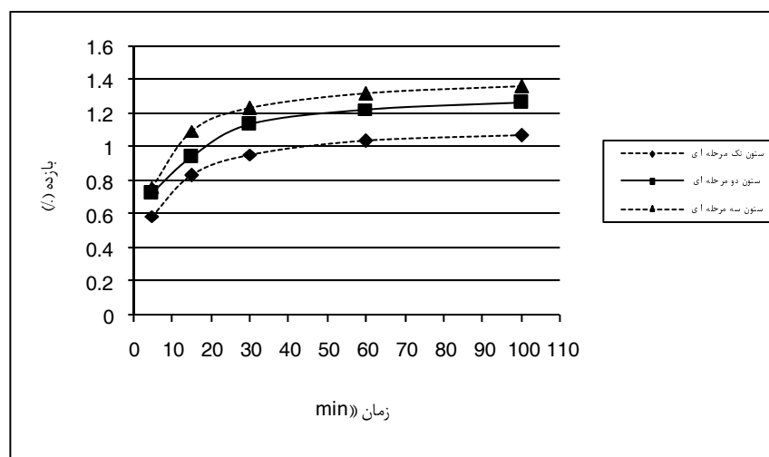
شکل شماره ۵- تغییرات بازده استخراج روغن فرار رزماری نسبت به افزایش تعداد مراحل برای شدت جریان حجمی بخار چهار لیتر بر دقیقه و جرم بستر ۱۰۰ گرم
