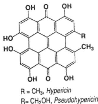
شکل شماره ۱- ساختمان شیمیایی هیپرسین و پزودوهیپرسین
