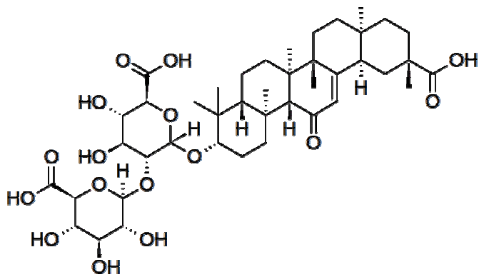
Fig. 1- Glycyrrhizin
