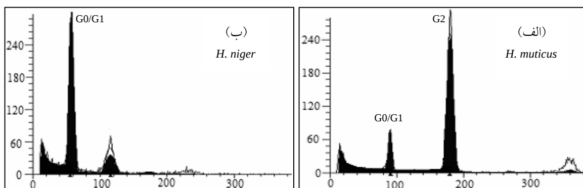
شکل شماره ۳- پروفیل فلوسایتومتری گیاهان بذرالبنج مصری (الف) در مقایسه با بذرالبنج سیاه (ب)
