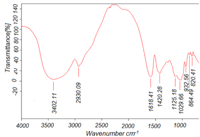
Fig. 2. Inulin FT-IR spectrum
