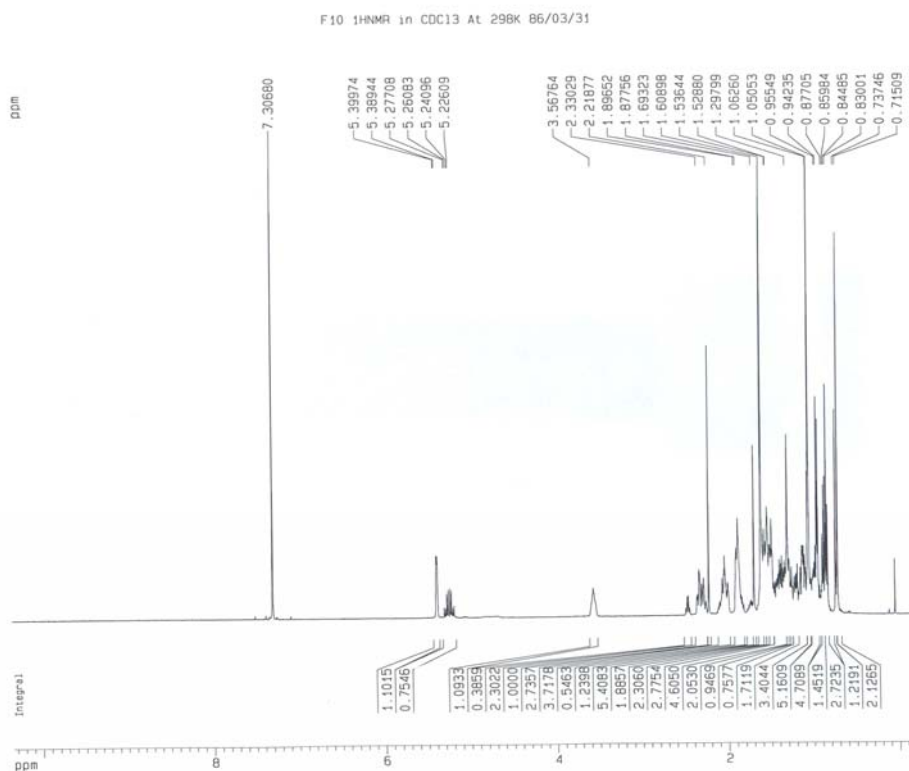
شکل شماره ۳- طیف ^1\text{H} NMR ترکیب \beta -استیگماسترول
