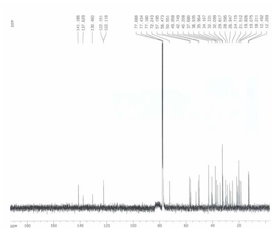
شکل شماره ۴- طیف ^{13}\text{C} NMR ترکیب \beta -استیگماسترول
