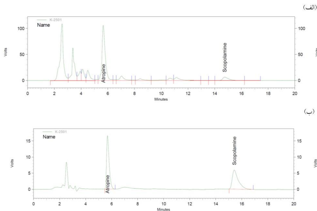
شکل شماره ۱- نمونه کروماتوگرام HPLC آتروپین و اسکوپولامین اندام گیاهی (الف) و محلول استاندارد (ب)
