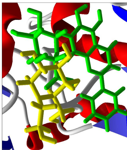
شکل ۳. موقعیت قرارگیری نویلنتین (ترکیب با رنگ سبز) و میگلنیتول (ترکیب با رنگ زرد) در جایگاه فعال آنزیم آلفاگلوکوزیداز و میزان هم‌پوشانی دو مولکول
