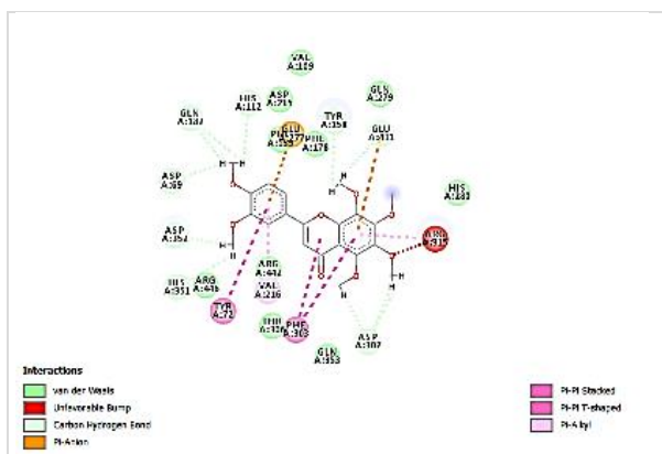
شکل ۲. بررسی اسیدهای آمینه در گیر در نویبلتین (چپ) و میگلیتول (راست) با آنزیم آلفاگلوکوزیداز توسط نرم افزار MVV (خط چین آبی؛ باندهای هیدروژن، خط چین قرمز؛ انتراکشن های الکترواستاتیک)
